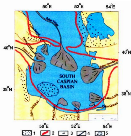
Рис. 1. Русла рек и дельтовые системы в бассейне Каспийского моря раннего плиоцена. 1 — относительные поднятия; 2 — пределы бассейна; 3 — русла рек; 4 — большие русла рек и подводные овраги; 5 — дельта [58., с.523-533].
