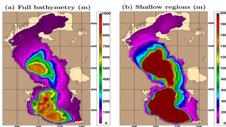
Рис. 4. Батиметрические карты Каспийского моря [International Tectonic Map of the Caspian Sea Region, 2005. V. Khain & N. Bogdanov (eds.). 96., с. 90].
