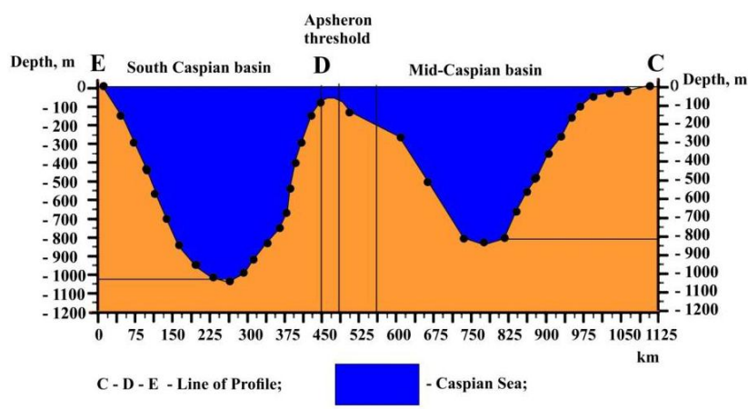
Рис. 5. Батиметрический профиль через Каспийское море по линии E-D-C (составил Э.Н. Халилов) [96., с. 94].
