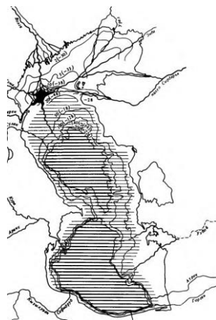
Рис. 2. Каспий при уровнях –48 (тонкая штриховка) и –168 (жирная штриховка) м абс. [79., с.130].
