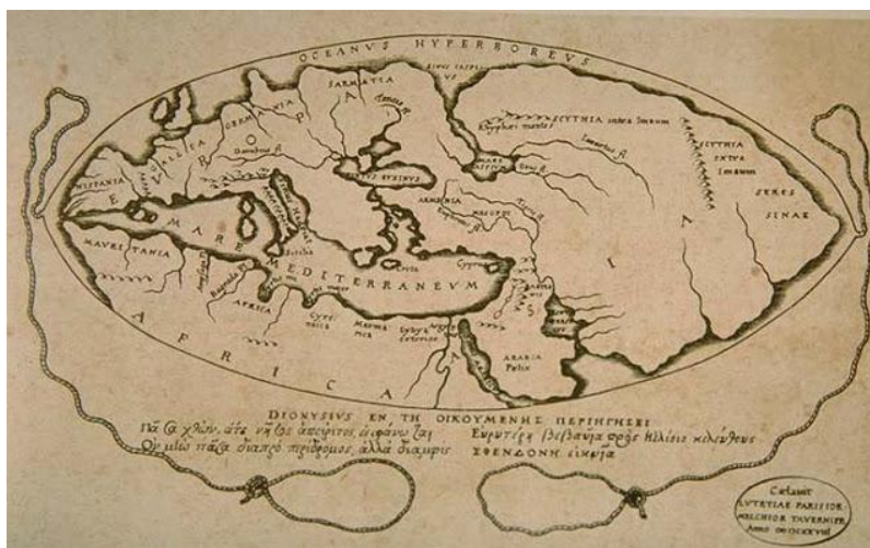
Рис. 6. Карта в соответствии с идеями греческого философа Посидония (139/135 – 51/50 гг. до н.э.). Карта изготовлена картографами Petrus Bertius и Melchior Tavernier в 1628 г. Многие детали не были известны Посидонию, но картографы показали идеи древнегреческого философа о расположении континентов. https://gorbutovich.livejournal.com/15890.html
